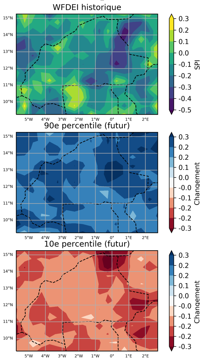
Figure 9: Ces cartes illustrent la projection multi-modèles pour la variation absolue de l'indice normalisé de précipitations, pour la période entre 2040 et 2059 (par rapport à la période de référence de 1950 à 2000) pour août. Elles indiquent les 90ème et 10ème percentiles de la distribution des modèles dans l'ensemble multi-modèles, calculés séparément en chaque point de grille, sur la région Burkina Faso. Ce diagramme montre la variation absolue pour le scénario RCP8.5.
