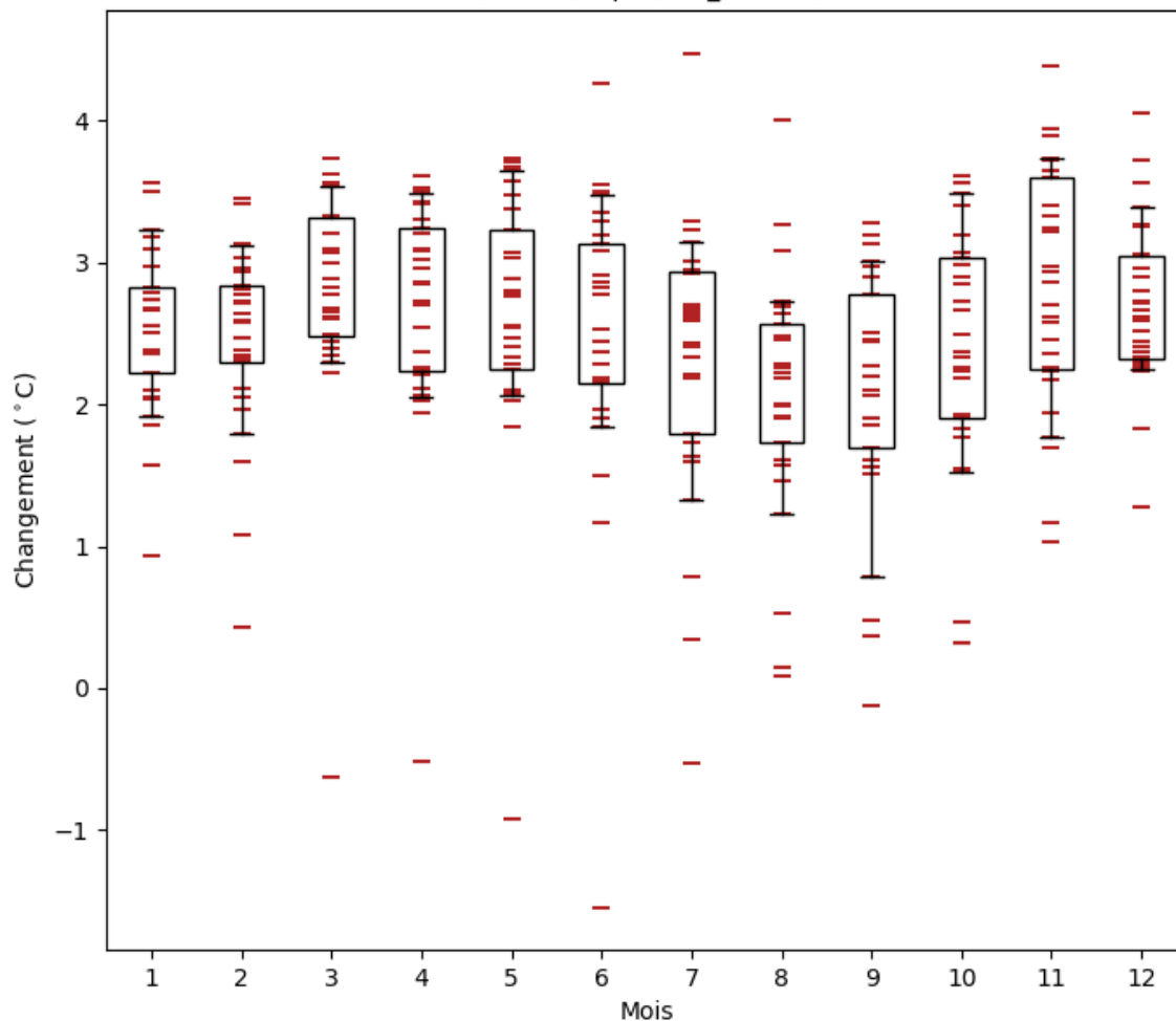
Burkina Faso : Changements de la moyenne climatologique mensuelle de Température Moyenne Journalière (Annuel ; rcp85; BC_0.5x0.5)
