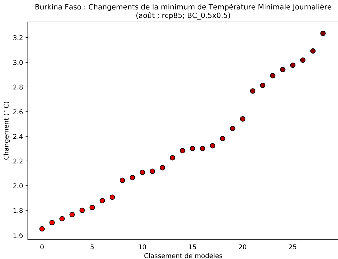
Figure 40: Ce diagramme de dispersion illustre la variation absolue de la minimum de température minimale journalière entre 2040 et 2059 (par rapport à la période de référence de 1950 à 2000) pour août. Chaque point indique la moyenne spatiale d'un modèle sur Burkina Faso; les points sont organisés ("rank", sur l'axe des abscisses) en fonction de la magnitude de leur valeur sur l'axe des ordonnées. Ce diagramme montre la variation absolue pour le scénario RCP8.5.
