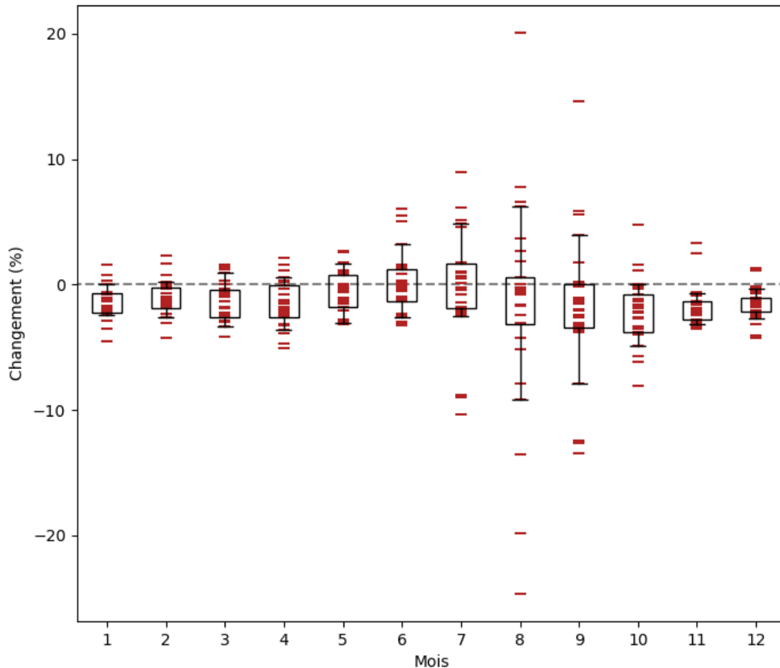
Burkina Faso : Changements (%) de la moyenne climatologique mensuelle de Flux Solaire Entrant À La Surface (Annuel ; rcp85; BC_0.5x0.5)
