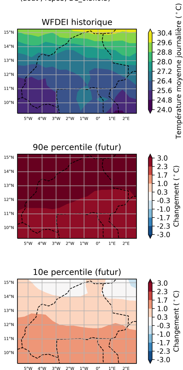
Figure 45: Ces cartes illustrent la projection multi-modèles pour la variation absolue de la moyenne de température moyenne journalière, pour la période entre 2040 et 2059 (par rapport à la période de référence de 1950 à 2000) pour août. Elles indiquent les 90ème et 10ème percentiles de la distribution des modèles dans l'ensemble multi-modèles, calculés séparément en chaque point de grille, sur la région Burkina Faso. Ce diagramme montre la variation absolue pour le scénario RCP8.5.
