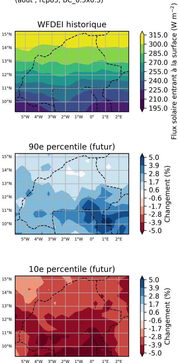
Figure 33: Ces cartes illustrent la projection multi-modèles pour du pourcentage de variation du maximum de flux solaire entrant à la surface, pour la période entre 2040 et 2059 (par rapport à la période de référence de 1950 à 2000) pour août. Elles indiquent les 90ème et 10ème percentiles de la distribution des modèles dans l'ensemble multi-modèles, calculés séparément en chaque point de grille, sur la région Burkina Faso. Ce diagramme montre le pourcentage de variation pour le scénario RCP8.5.
