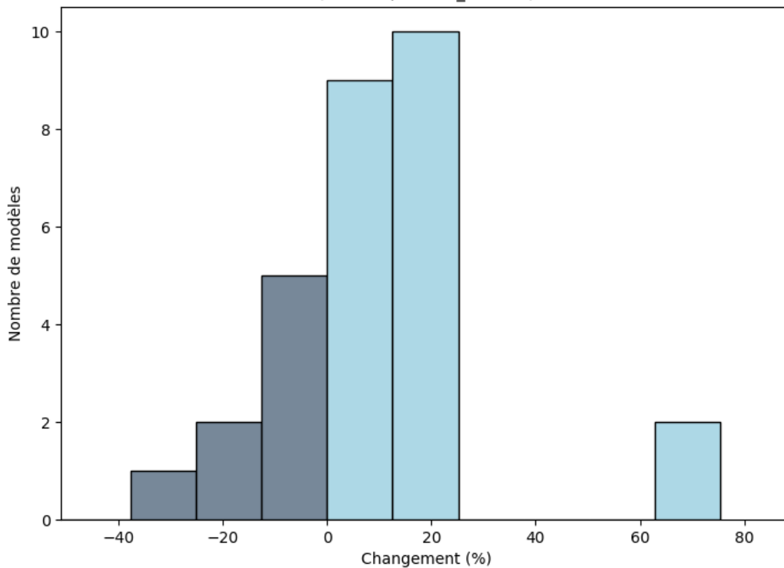
Burkina Faso: Changements (%) du maximum de précipitations totales sur une période de 5 jours (août; rcp85; BC_0.5x0.5)
