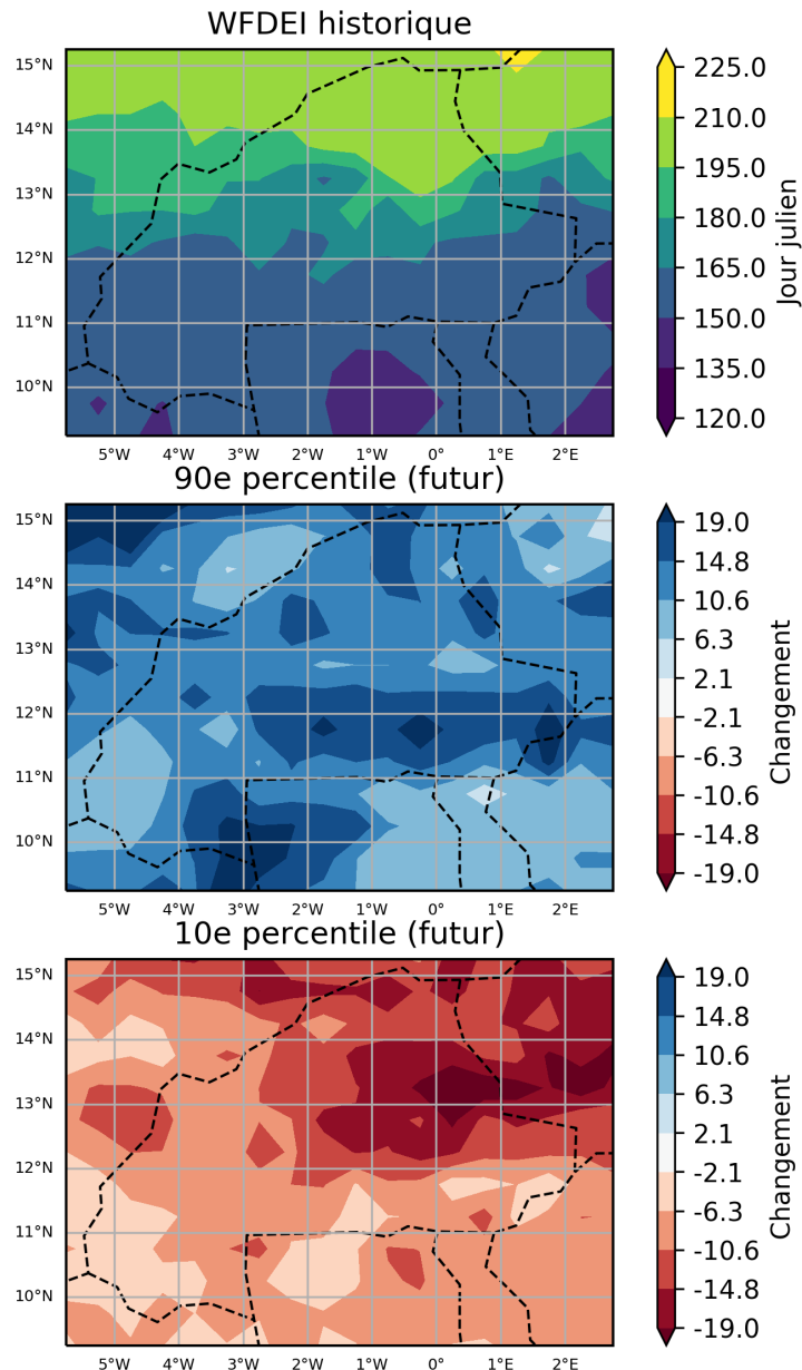
Figure 5: Ces cartes illustrent la projection multi-modèles pour la variation absolue de la date de déclenchement de la mousson (Marteau), pour la période entre 2040 et 2059 (par rapport à la période de référence de 1950 à 2000) pour mai à septembre. Elles indiquent les 90ème et 10ème percentiles de la distribution des modèles dans l'ensemble multi-modèles, calculés séparément en chaque point de grille, sur la région Burkina Faso. Ce diagramme montre la variation absolue pour le scénario RCP8.5.
