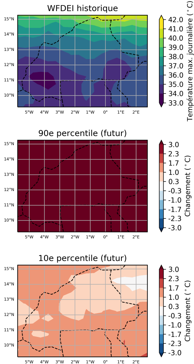
Figure 29: Ces cartes illustrent la projection multi-modèles pour la variation absolue du maximum de température maximale journalière, pour la période entre 2040 et 2059 (par rapport à la période de référence de 1950 à 2000) pour août. Elles indiquent les 90ème et 10ème percentiles de la distribution des modèles dans l'ensemble multi-modèles, calculés séparément en chaque point de grille, sur la région Burkina Faso. Ce diagramme montre la variation absolue pour le scénario RCP8.5.
