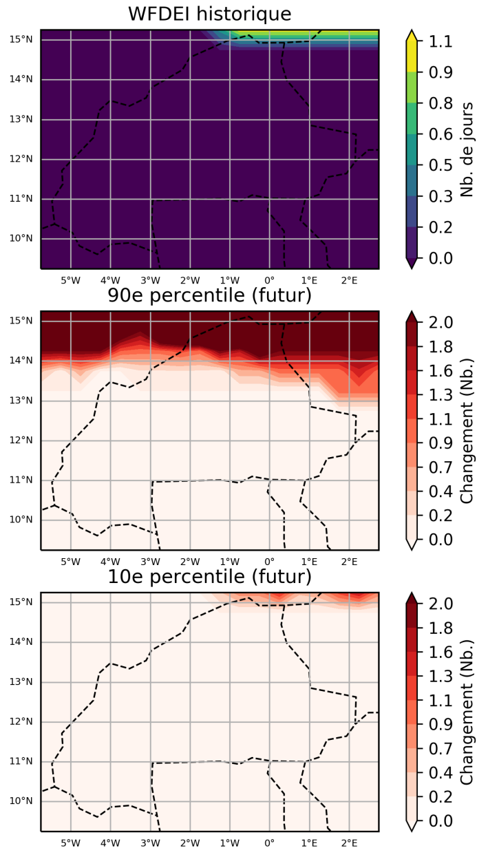
Figure 68: Ces cartes illustrent la projection multi-modèles pour la variation absolue du nombre de jours avec une température maximale > 40^{\circ}\text{C} , pour la période entre 2040 et 2059 (par rapport à la période de référence de 1950 à 2000) pour août. Elles indiquent les 90ème et 10ème percentiles de la distribution des modèles dans l'ensemble multi-modèles, calculés séparément en chaque point de grille, sur la région Burkina Faso. Ce diagramme montre la variation absolue pour le scénario RCP8.5.
