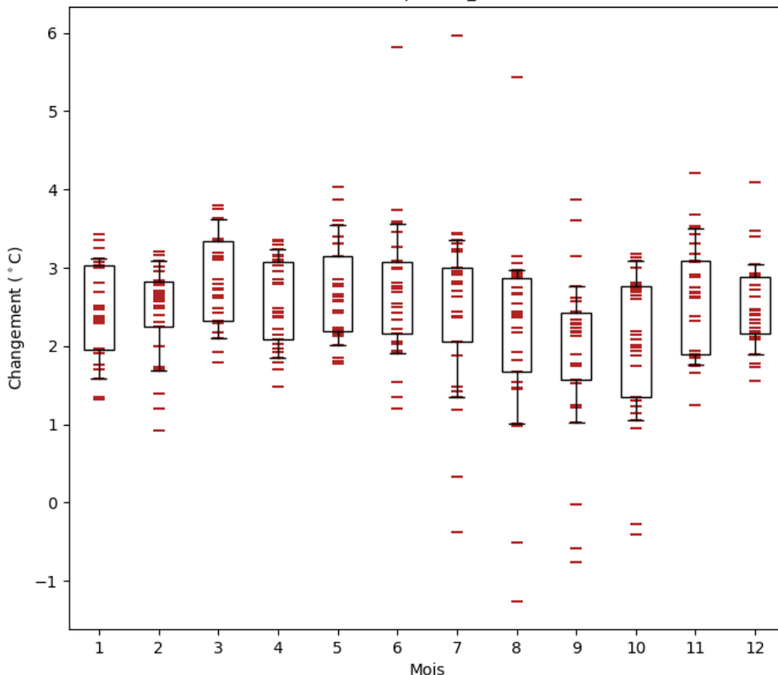
Burkina Faso : Changements de la moyenne climatologique mensuelle de Température Maximale Journalière (Annuel ; rcp85; BC_0.5x0.5)
