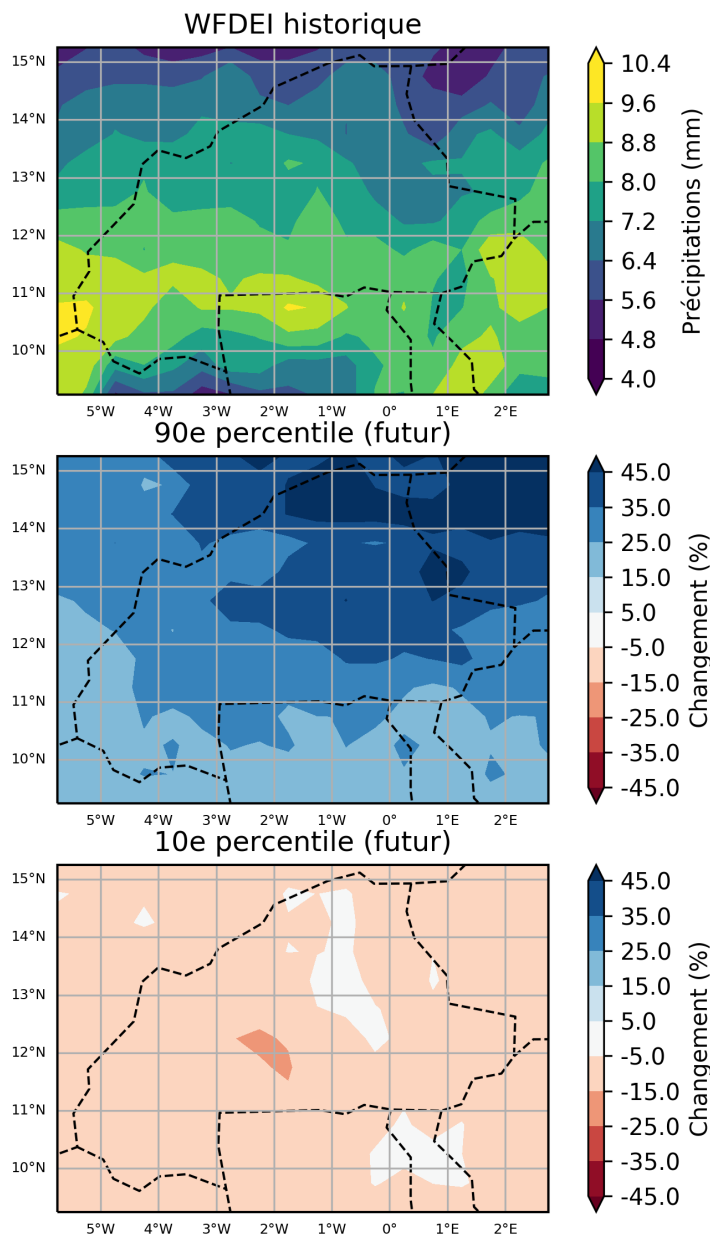
Figure 53: Ces cartes illustrent la projection multi-modèles pour du pourcentage de variation des précipitations moyennes par jour pluvieux, pour la période entre 2040 et 2059 (par rapport à la période de référence de 1950 à 2000) pour août. Elles indiquent les 90ème et 10ème percentiles de la distribution des modèles dans l'ensemble multi-modèles, calculés séparément en chaque point de grille, sur la région Burkina Faso. Ce diagramme montre le pourcentage de variation pour le scénario RCP8.5.
