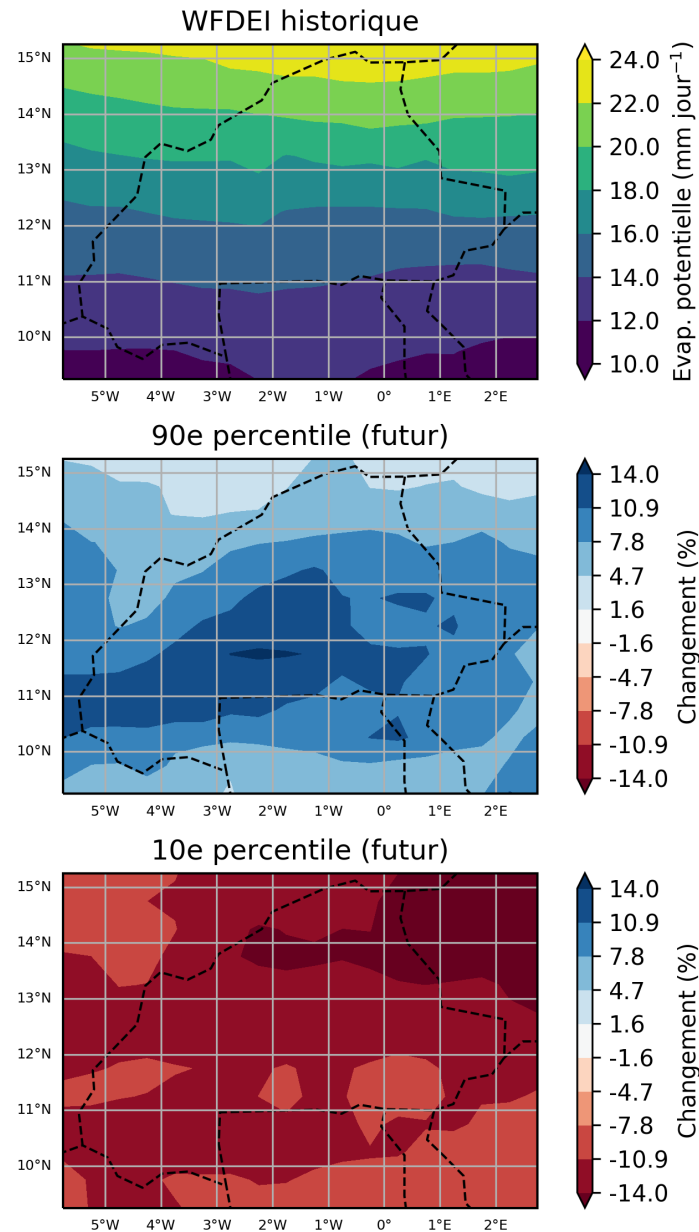
Figure 1: Ces cartes illustrent la projection multi-modèles pour du pourcentage de variation de l'évapotranspiration potentielle, pour la période entre 2040 et 2059 (par rapport à la période de référence de 1950 à 2000) pour août. Elles indiquent les 90ème et 10ème percentiles de la distribution des modèles dans l'ensemble multi-modèles, calculés séparément en chaque point de grille, sur la région Burkina Faso. Ce diagramme montre le pourcentage de variation pour le scénario RCP8.5.
