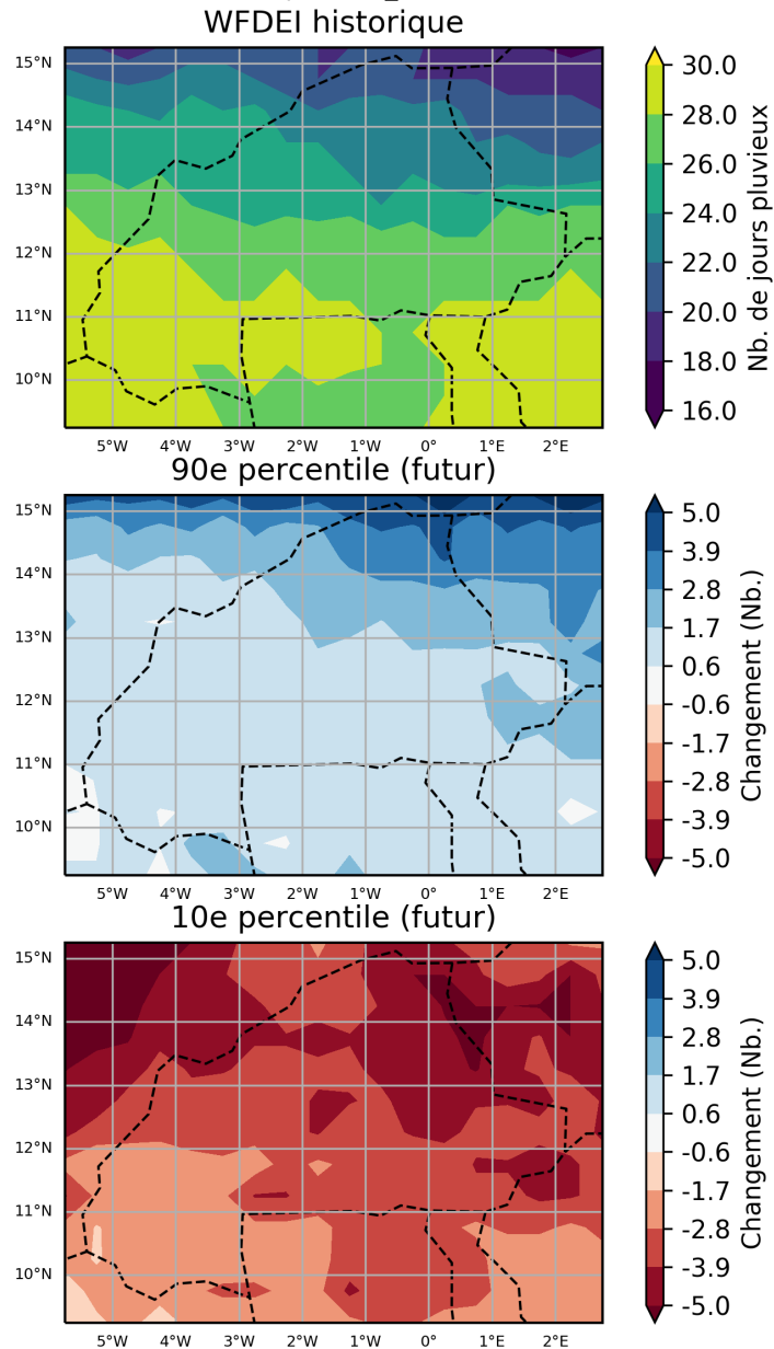
Figure 64: Ces cartes illustrent la projection multi-modèles pour la variation absolue du nombre de jours pluvieux ( >1 \text{ mm jour}^{-1} ), pour la période entre 2040 et 2059 (par rapport à la période de référence de 1950 à 2000) pour août. Elles indiquent les 90ème et 10ème percentiles de la distribution des modèles dans l'ensemble multi-modèles, calculés séparément en chaque point de grille, sur la région Burkina Faso. Ce diagramme montre la variation absolue pour le scénario RCP8.5.
