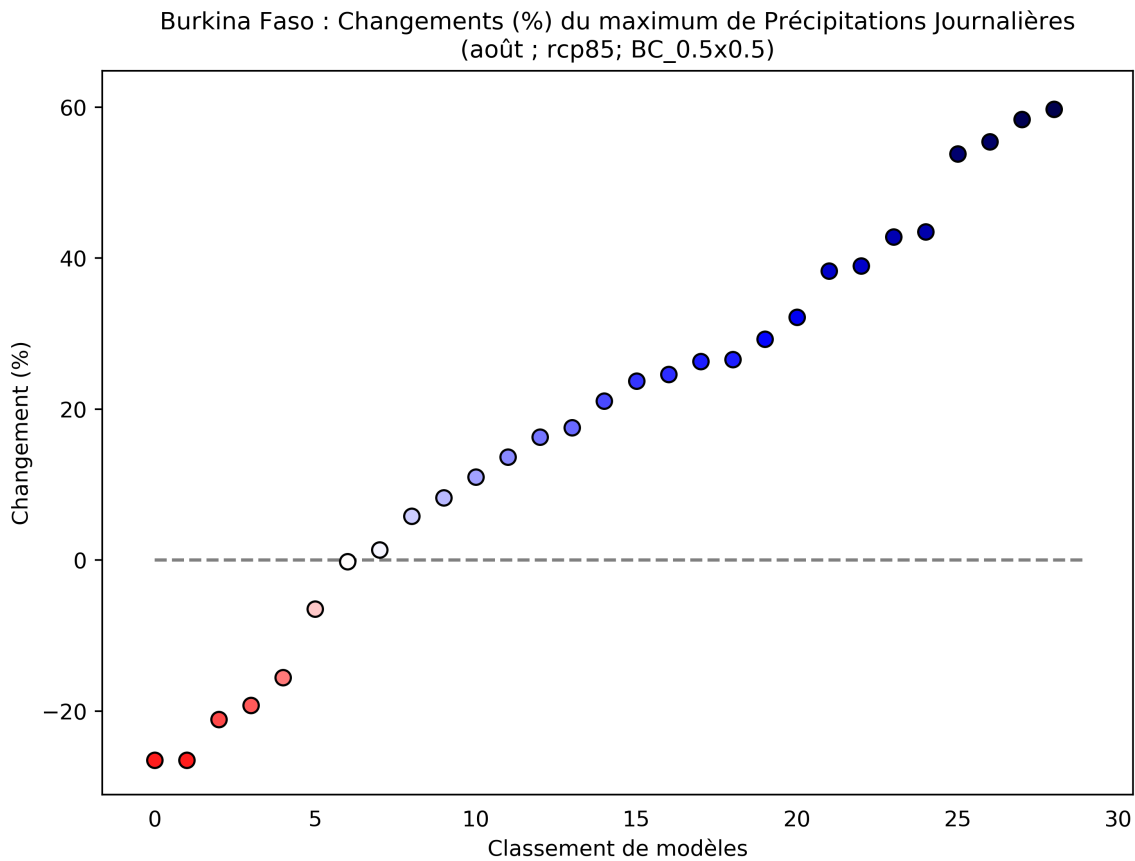
Figure 28: Ce diagramme de dispersion illustre du pourcentage de variation du maximum de précipitations journalières entre 2040 et 2059 (par rapport à la période de référence de 1950 à 2000) pour août. Chaque point indique la moyenne spatiale d'un modèle sur Burkina Faso; les points sont organisés ("rank", sur l'axe des abscisses) en fonction de la magnitude de leur valeur sur l'axe des ordonnées. Ce diagramme montre le pourcentage de variation pour le scénario RCP8.5.
