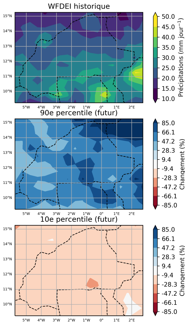
Figure 25: Ces cartes illustrent la projection multi-modèles pour du pourcentage de variation du maximum de précipitations journalières, pour la période entre 2040 et 2059 (par rapport à la période de référence de 1950 à 2000) pour août. Elles indiquent les 90ème et 10ème percentiles de la distribution des modèles dans l'ensemble multi-modèles, calculés séparément en chaque point de grille, sur la région Burkina Faso. Ce diagramme montre le pourcentage de variation pour le scénario RCP8.5.
