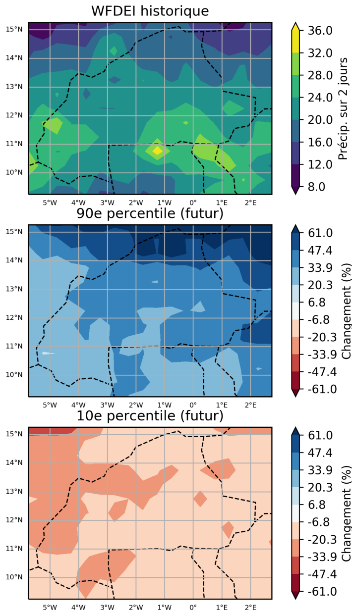
Figure 88: Ces cartes illustrent la projection multi-modèles pour du pourcentage de variation du maximum de précipitations totales sur une période de 2 jours, pour la période entre 2040 et 2059 (par rapport à la période de référence de 1950 à 2000) pour août. Elles indiquent les 90ème et 10ème percentiles de la distribution des modèles dans l'ensemble multi-modèles, calculés séparément en chaque point de grille, sur la région Burkina Faso. Ce diagramme montre le pourcentage de variation pour le scénario RCP8.5.
