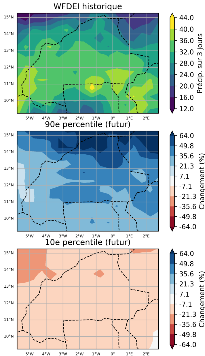
Figure 84: Ces cartes illustrent la projection multi-modèles pour du pourcentage de variation du maximum de précipitations totales sur une période de 3 jours, pour la période entre 2040 et 2059 (par rapport à la période de référence de 1950 à 2000) pour août. Elles indiquent les 90ème et 10ème percentiles de la distribution des modèles dans l'ensemble multi-modèles, calculés séparément en chaque point de grille, sur la région Burkina Faso. Ce diagramme montre le pourcentage de variation pour le scénario RCP8.5.
