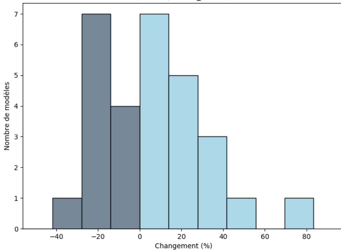
Burkina Faso: Changements (%) du maximum de précipitations totales sur une période de 2 jours (août; rcp85; BC_0.5x0.5)
