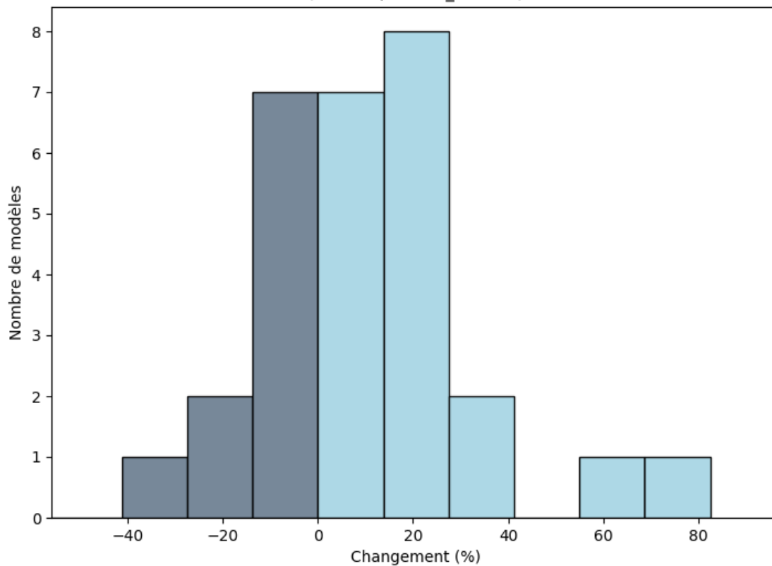
Burkina Faso: Changements (%) du maximum de précipitations totales sur une période de 3 jours (août; rcp85; BC_0.5x0.5)
