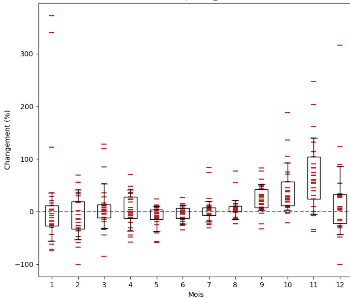
Burkina Faso : Changements (%) de la moyenne climatologique mensuelle de Précipitations Journalières (Annuel ; rcp85; BC_0.5x0.5)
