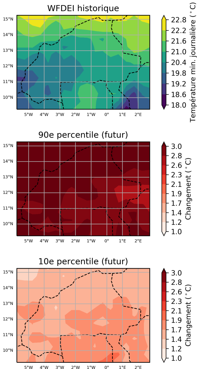
Figure 37: Ces cartes illustrent la projection multi-modèles pour la variation absolue de la minimum de température minimale journalière, pour la période entre 2040 et 2059 (par rapport à la période de référence de 1950 à 2000) pour août. Elles indiquent les 90ème et 10ème percentiles de la distribution des modèles dans l'ensemble multi-modèles, calculés séparément en chaque point de grille, sur la région Burkina Faso. Ce diagramme montre la variation absolue pour le scénario RCP8.5.
