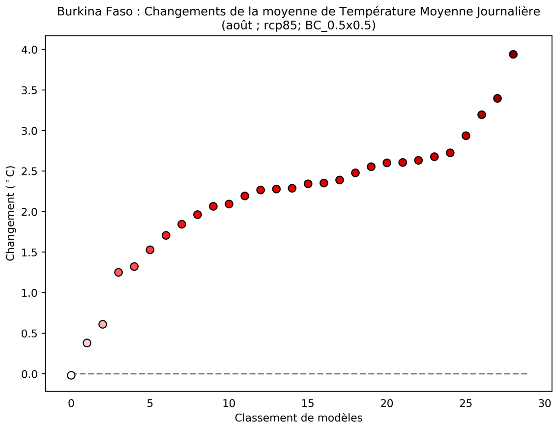
Figure 48: Ce diagramme de dispersion illustre la variation absolue de la moyenne de température moyenne journalière entre 2040 et 2059 (par rapport à la période de référence de 1950 à 2000) pour août. Chaque point indique la moyenne spatiale d'un modèle sur Burkina Faso; les points sont organisés ("rank", sur l'axe des abscisses) en fonction de la magnitude de leur valeur sur l'axe des ordonnées. Ce diagramme montre la variation absolue pour le scénario RCP8.5.
