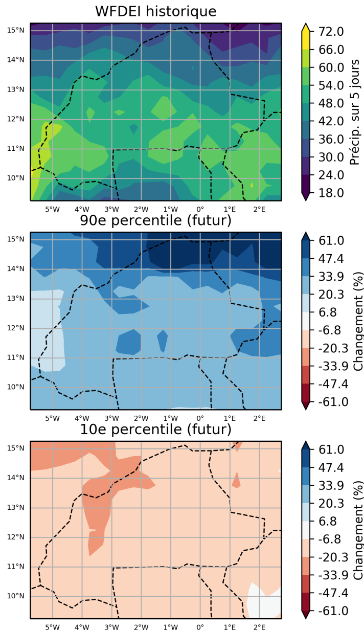
Figure 80: Ces cartes illustrent la projection multi-modèles pour du pourcentage de variation du maximum de précipitations totales sur une période de 5 jours, pour la période entre 2040 et 2059 (par rapport à la période de référence de 1950 à 2000) pour août. Elles indiquent les 90ème et 10ème percentiles de la distribution des modèles dans l'ensemble multi-modèles, calculés séparément en chaque point de grille, sur la région Burkina Faso. Ce diagramme montre le pourcentage de variation pour le scénario RCP8.5.
