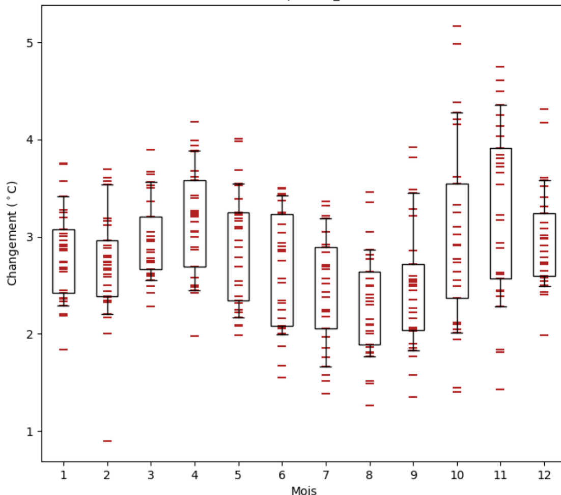
Burkina Faso : Changements de la moyenne climatologique mensuelle de Température Minimale Journalière (Annuel ; rcp85; BC_0.5x0.5)
