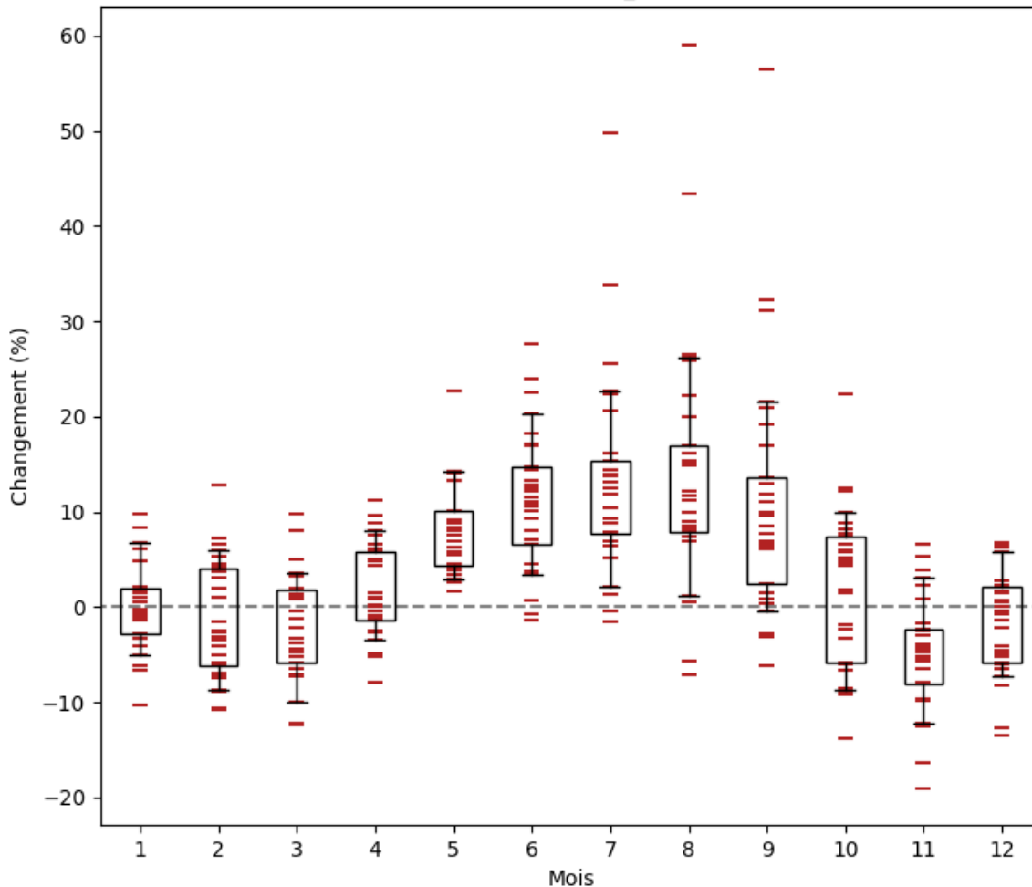
Burkina Faso : Changements (%) de la moyenne climatologique mensuelle de Vitesse Du Vent Près De La Surface (Annuel ; rcp85; BC_0.5x0.5)
