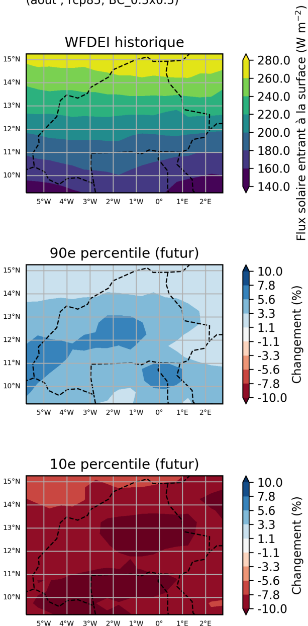
Figure 49: Ces cartes illustrent la projection multi-modèles pour du pourcentage de variation de la moyenne de flux solaire entrant à la surface, pour la période entre 2040 et 2059 (par rapport à la période de référence de 1950 à 2000) pour août. Elles indiquent les 90ème et 10ème percentiles de la distribution des modèles dans l'ensemble multi-modèles, calculés séparément en chaque point de grille, sur la région Burkina Faso. Ce diagramme montre le pourcentage de variation pour le scénario RCP8.5.
